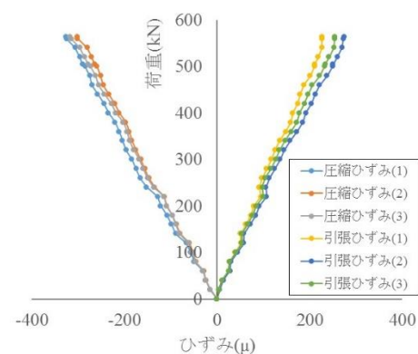
図 14 セン断試験体の荷重－ひずみ関係
