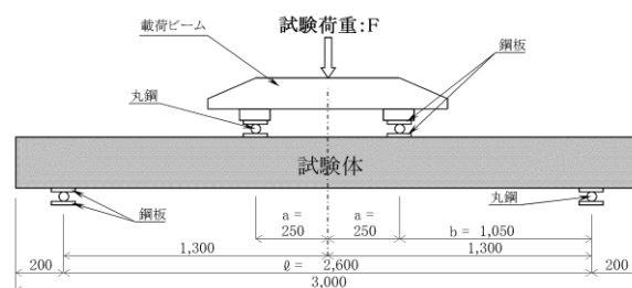
図 7 曲げ荷重試験模式図
