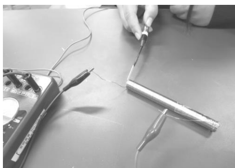
図2 磁束密度の測定の様子
