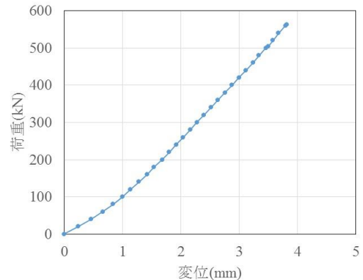
図 13 セン断試験体の荷重－変位関係 (中央のみ)
