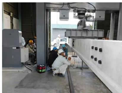
写真 3 曲げ載荷試験およびひび割れ観測 (BS12)
