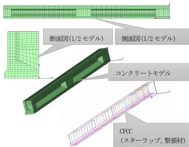
図 17 有限要素モデル
